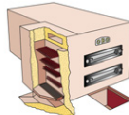
Four à chauffage indirect « Perkins »
