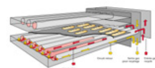
Four à double recyclage « Ambassador »
